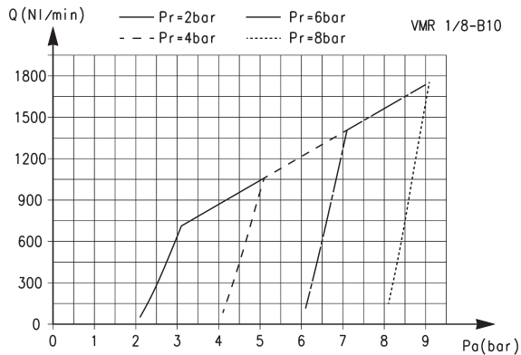
DIAGRAMMA DI PORTATA
