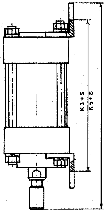
Пневмоцилиндр 1112-D-S
